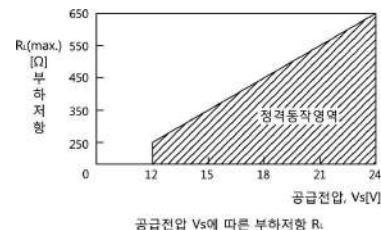
공급전압 V_s 에 따른 부하저항 R_L
